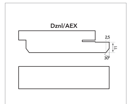
Verdekte Dznl-kantafwerking in de lengte van de plafondpanelen en vlakleg in de breedte.
